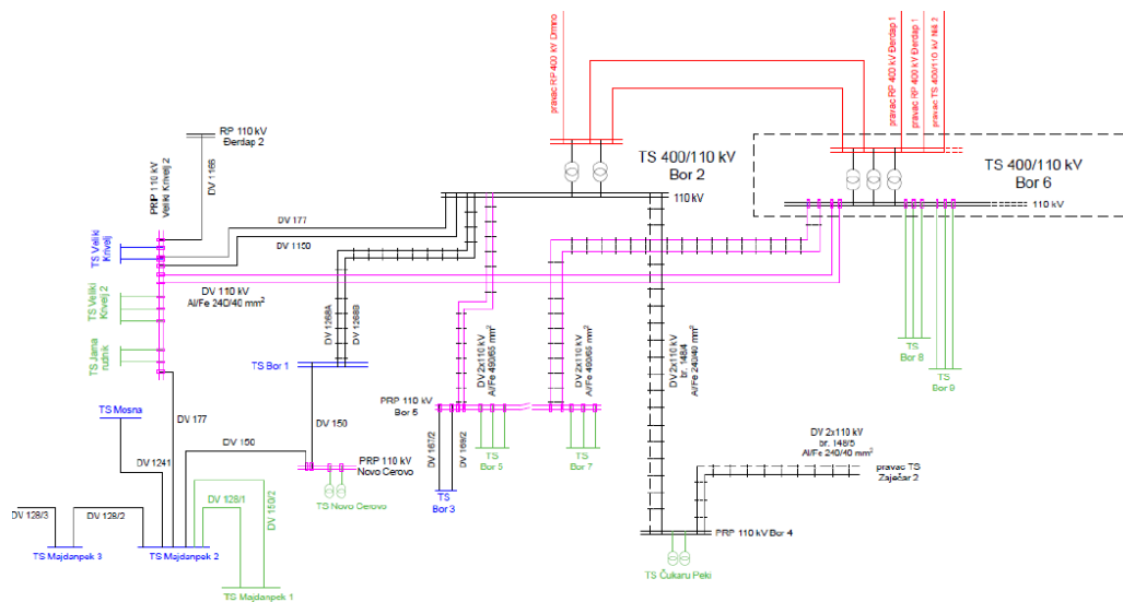
Slika 2. Šema uklapanja TS 110/10 kV Bor 8 u EES
